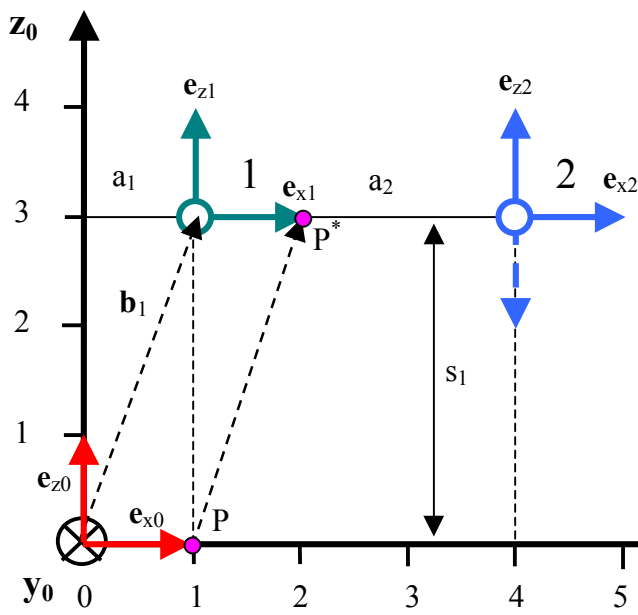
Bild 5.2: Gelenkarmschema
